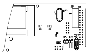
Рисунок 6.9 – Вид на разъем XP2
