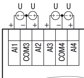
Рисунок 5.5 – Схема подключения активных датчиков с выходом типа «Напряжение 0...10 В»
