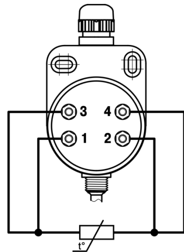
Рисунок Д.12 – Четырехпроводная схема подключения проводов к клеммам пластмассовой коммутационной головки ДТС 125Л с одним ЧЭ
