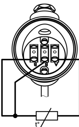
Рисунок Д.5 – Трехпроводная схема подключения проводов к клеммам металлической коммутационной головки с одним ЧЭ
