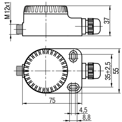
Рисунок В.5 – Увеличенная пластмассовая коммутационная головка
