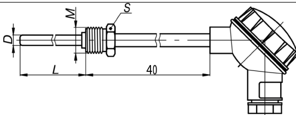
Рисунок Б.4 – Конструктивное исполнение 335
