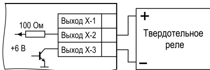
Рисунок 5.6 – Схема подключения к ВУ типа Т
