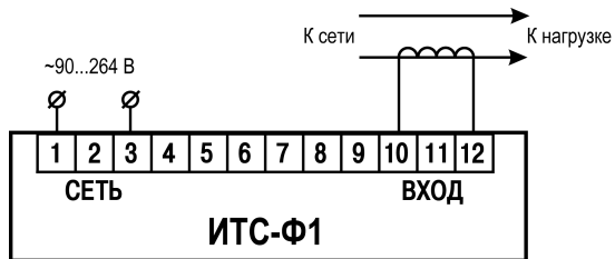
Рисунок 5.3 – Схема подключения с трансформатором
