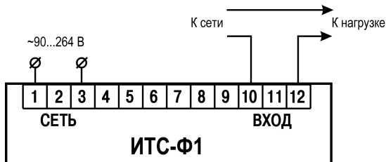
Рисунок 5.2 – Схема подключения без трансформатора
