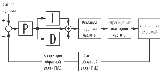
Рисунок 60 – работа ПИД-регулятора.
