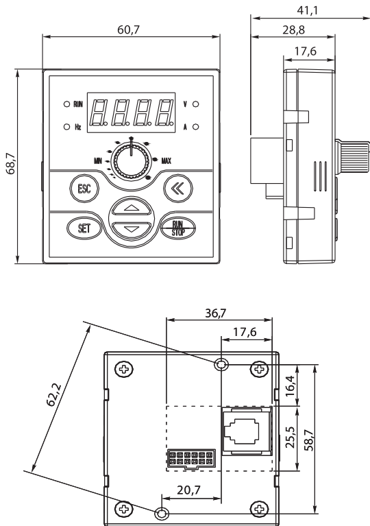
Рисунок 10 – габаритные и установочные размеры панели управления AFD-LPNL.11.
