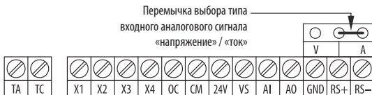
Рисунок 12 – Клеммы цепей управления.
