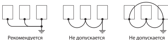
Рисунок 11 – рекомендуемая схема заземления нескольких ПЧ.
