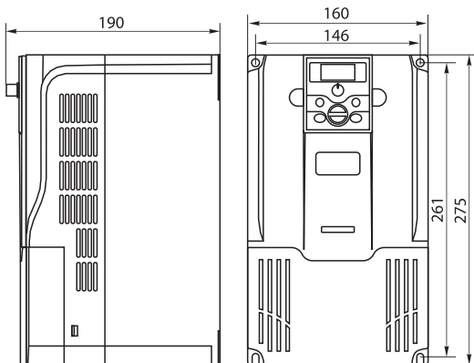
Габарит корпуса 5
