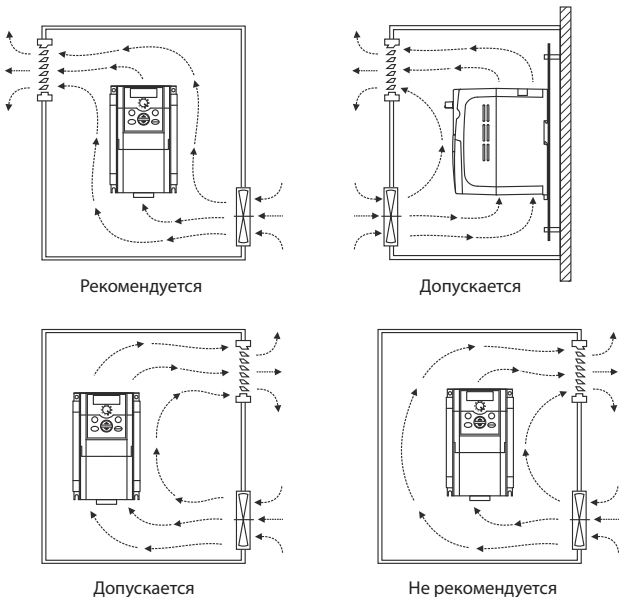
Рисунок 8 – Расположение элементов системы дополнительной вентиляции.
