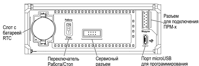
Рисунок 14 – Лицевая панель под крышкой
