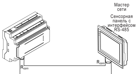
Рисунок 10 – Типовая схема подключения в режиме Slave
