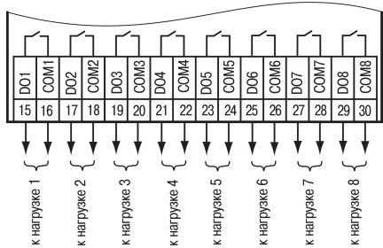
Рисунок 8 – Схема подключения нагрузки к ВЭ типа Р
