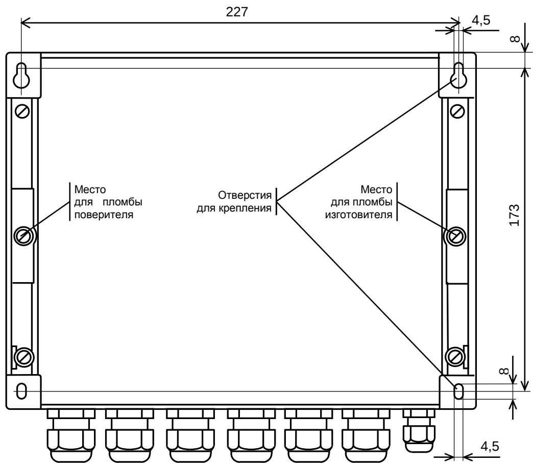
Рисунок 3.3 – Вид сзади
