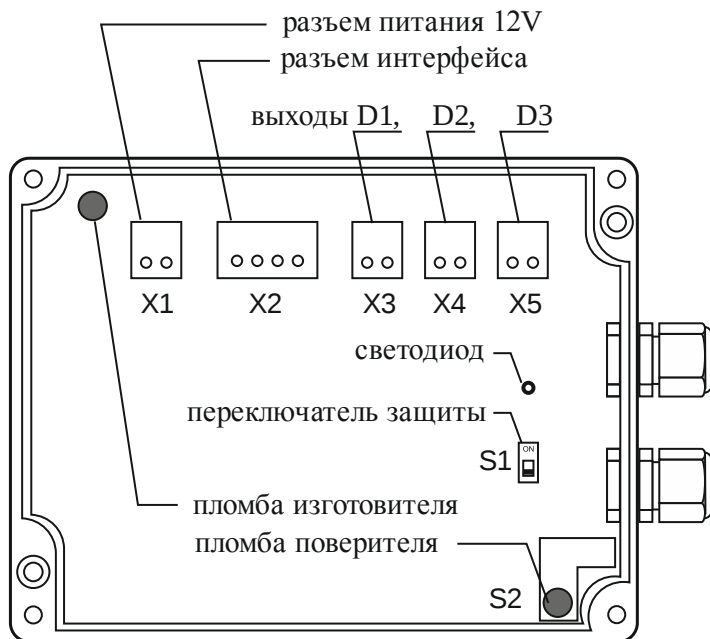
Рисунок 3.4 – Монтажный отсек
