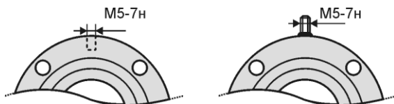
Рисунок 15. Доработка фланцев
