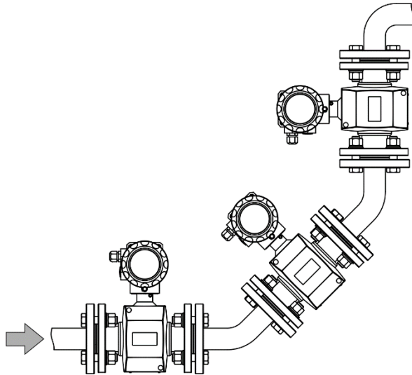
Рисунок 10. Рекомендуемые варианты установки
