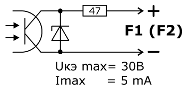
Рисунок 3. Схема выходного каскада
