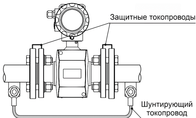
Рисунок 173. Подключение защитных и шунтирующего токопроводов
