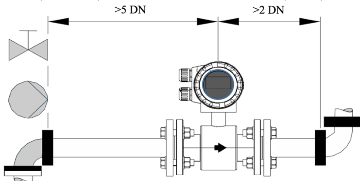
Рисунок 13. Требования к длине прямых участков
