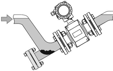
Рисунок 11. Установка расходомера в частично заполненном трубопроводе
