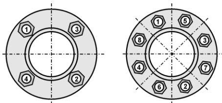
Рисунок 16. Порядок затяжки гаек
