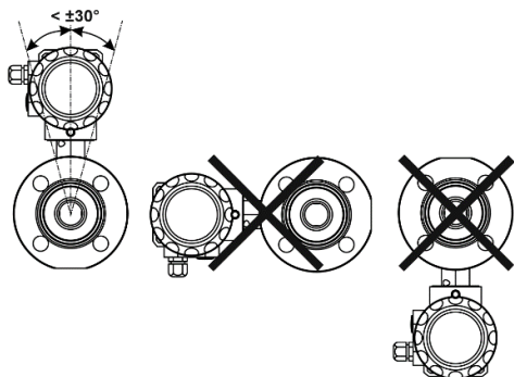
Рисунок 12. Установка на горизонтальных участках трубопровода
