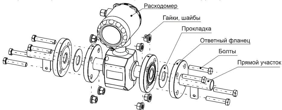
Рисунок 14. Установка расходомера
