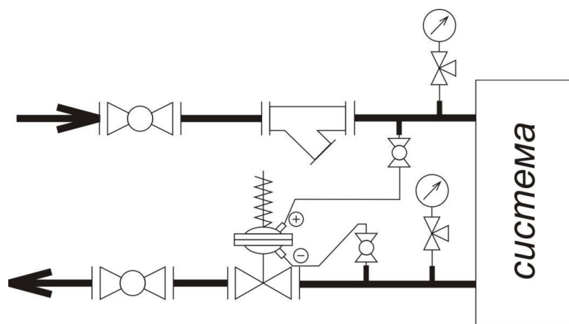
Регулятор перепада давления (установка – обратка)
