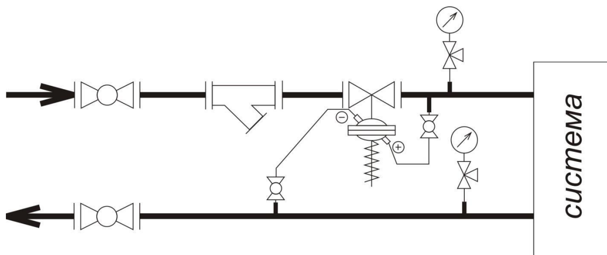
Регулятор перепада давления (установка – подача)
